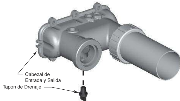
Fig. 22: Ubicacion del Tapon de Drenaje
