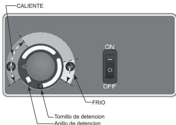
Fig. 17: Termostato De Temperatura Del Agua
