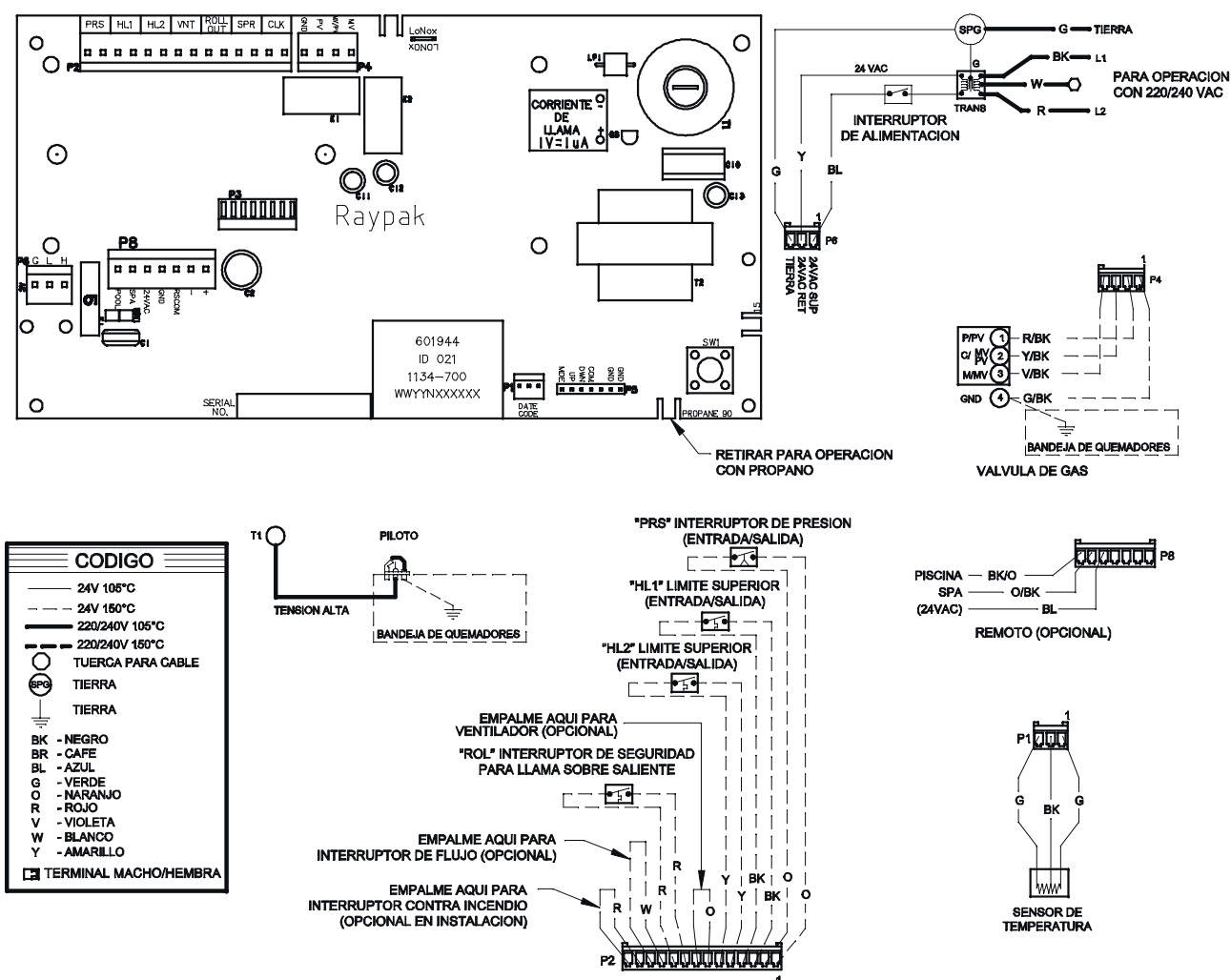
Fig. 21: Diagrama Electronico - Modelo 156 (Calentadores Fabricados Para Chile)
