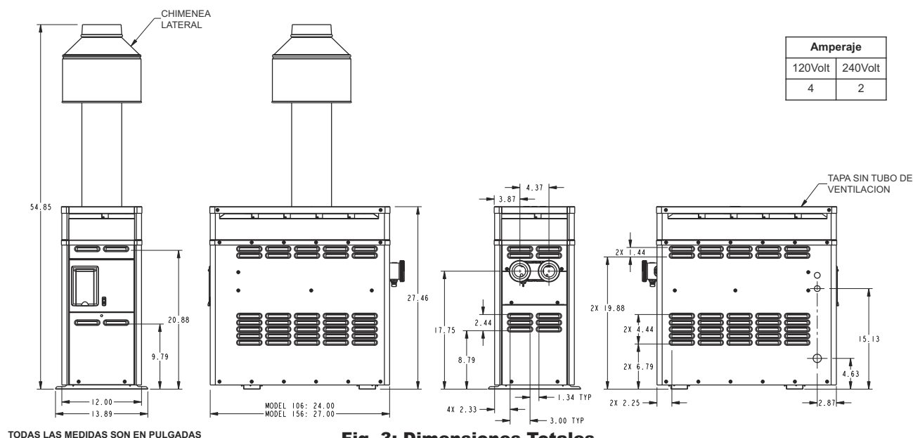
Fig. 3: Dimensiones Totales
