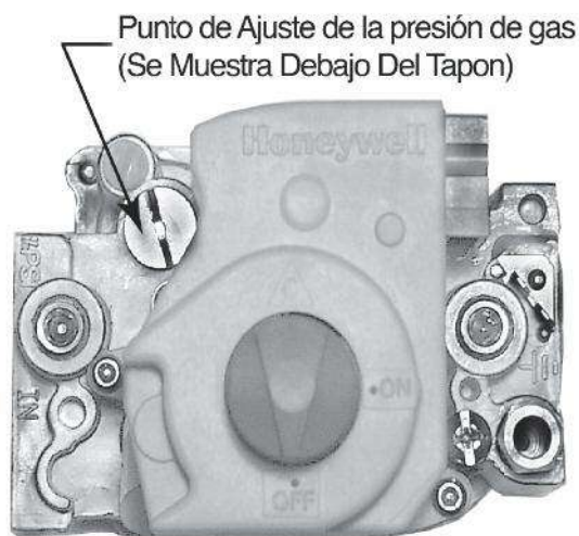
Válvula de Gas Honeywell
