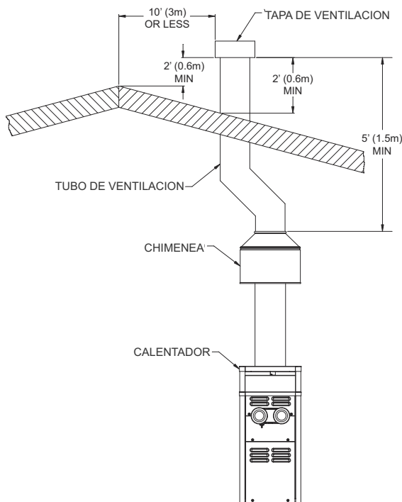
Fig. 6: Requerimientos para tubos de ventilación
